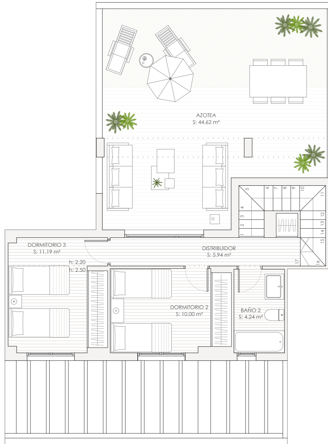
PLANTA BAJOCUBIERTA
