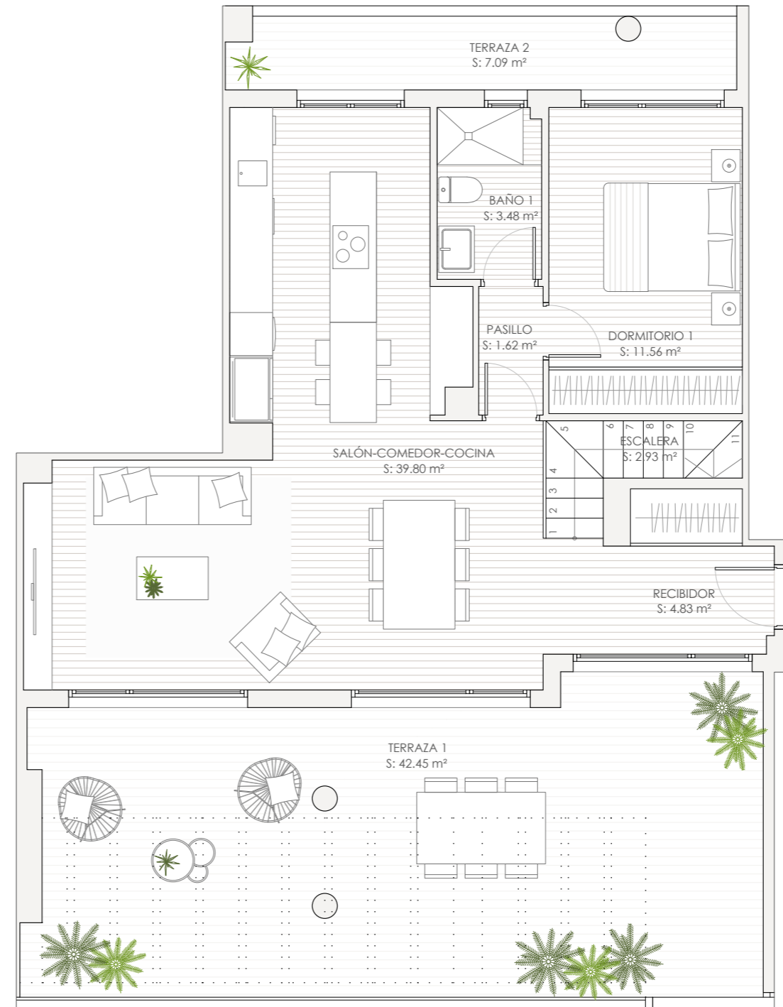
PLANTA 5ª
